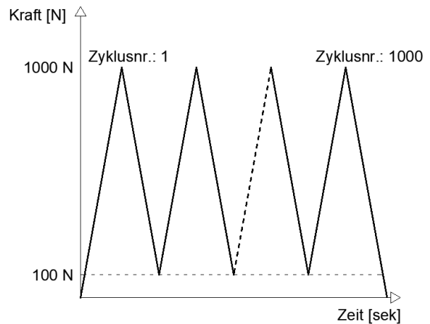
Abbildung 4: Kraft-Zeitdiagramm
