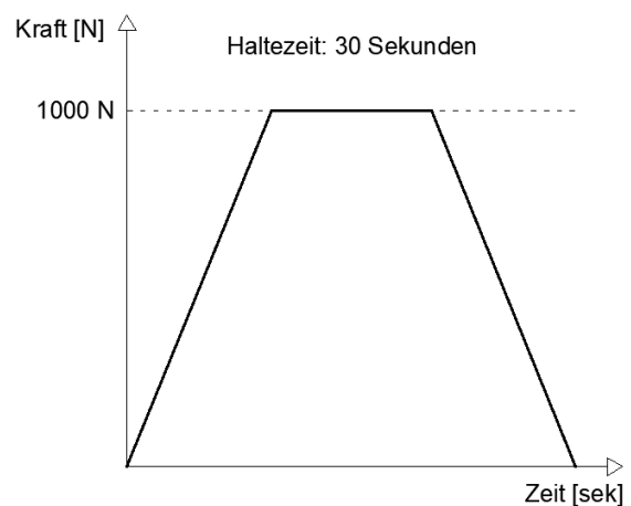
Abbildung 17: Kraft-Zeitdiagramm
