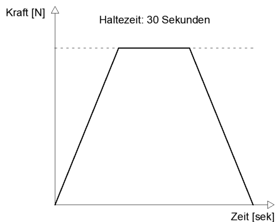
Abbildung 14: Kraft-Zeitdiagramm
