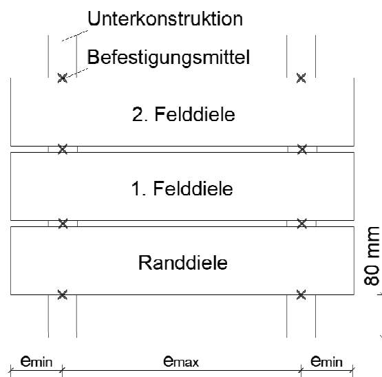
Abbildung 1: Schematische Darstellung eines Prüfkörpers
