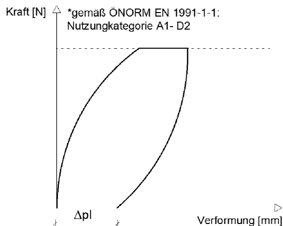
Abbildung 6: Kraft-Verformungsdiagramm
